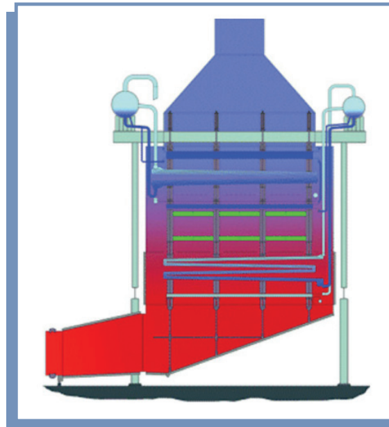
Ilustración 6. Caldera HRSG (vertical). Fuente: Curso - Centrales Térmicas de Ciclo Combinado (renovetc)
