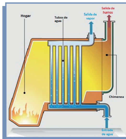
Ilustración 5. Caldera ACUOTUBULAR. Fuente: How Stuff Works (2008)
