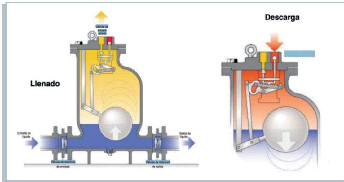
Ilustración 15. Funcionamiento de bomba de condensado mecánica. Fuente: Spirax Sarco
