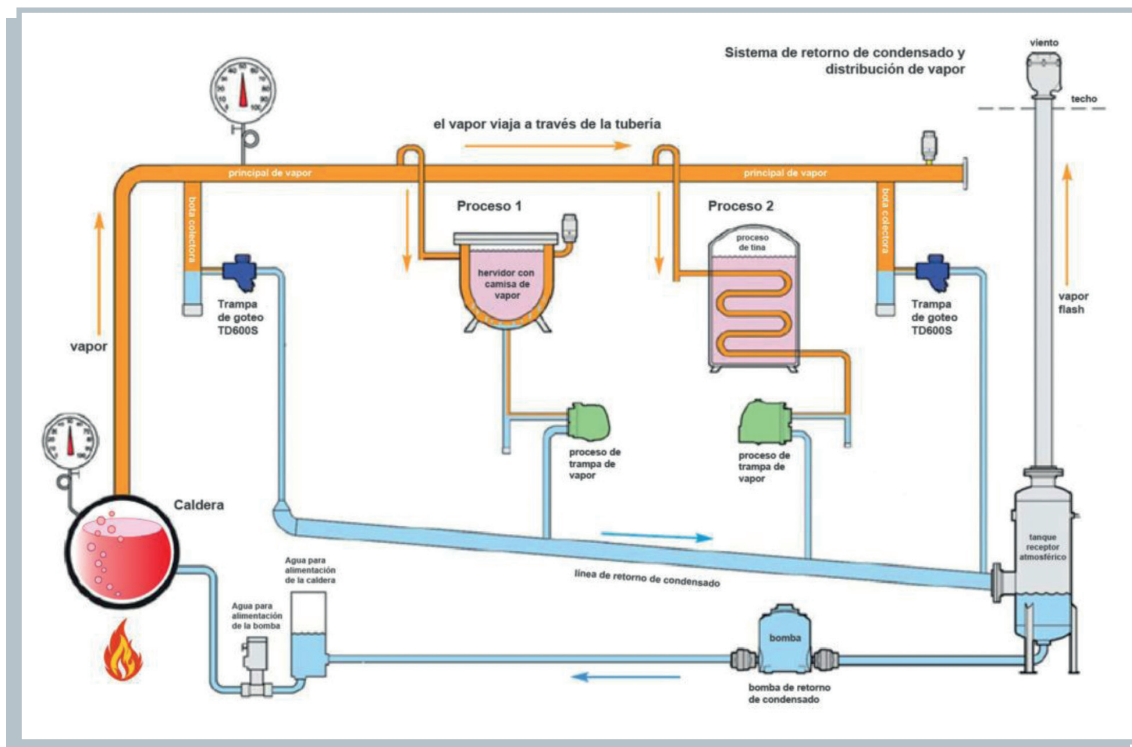
Ilustración 14. Sistema general de vapor con sistema de condensado.
