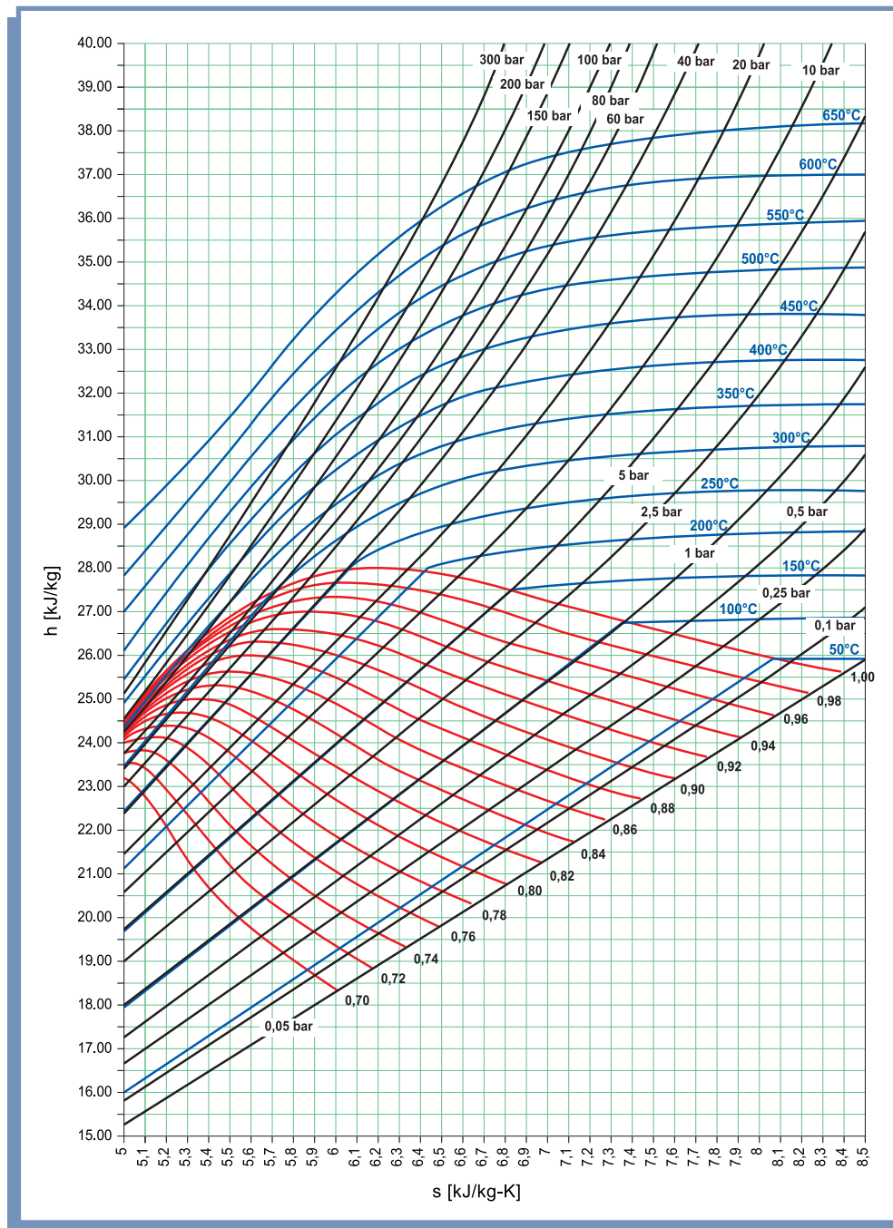
Ilustración 24 Diagrama de Mollier. Fuente Academia (Mar Cledera Castro)
