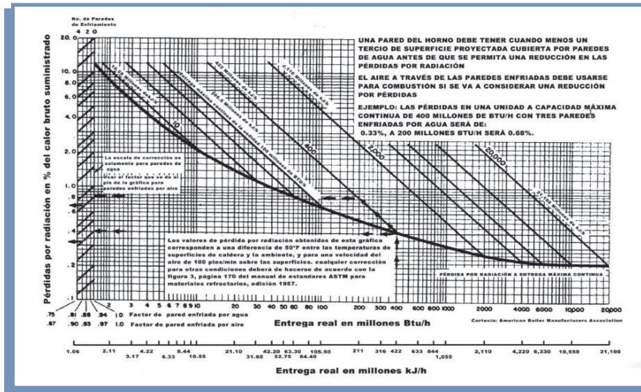
Ilustración 25. Pérdidas por radiación. Fuente: Norma ASME.
