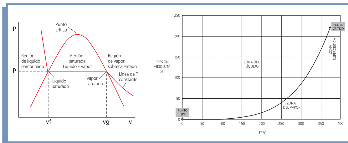
Ilustración 3. Diagramas P-T y P-v para el agua. Fuente: Moran & Shapiro; "Termodinámica".
