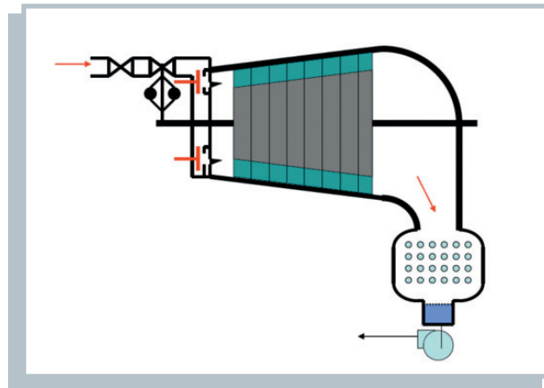
Ilustración 20. TV de condensación. Fuente: US DOE Steam BestPractices End User Training.
