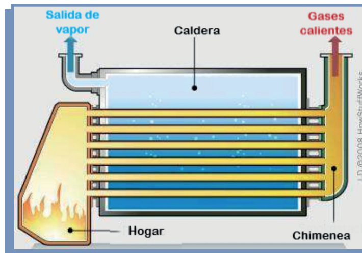
Ilustración 4. Caldera HUMOTUBULAR. Fuente: How Stuff Works (2008)
