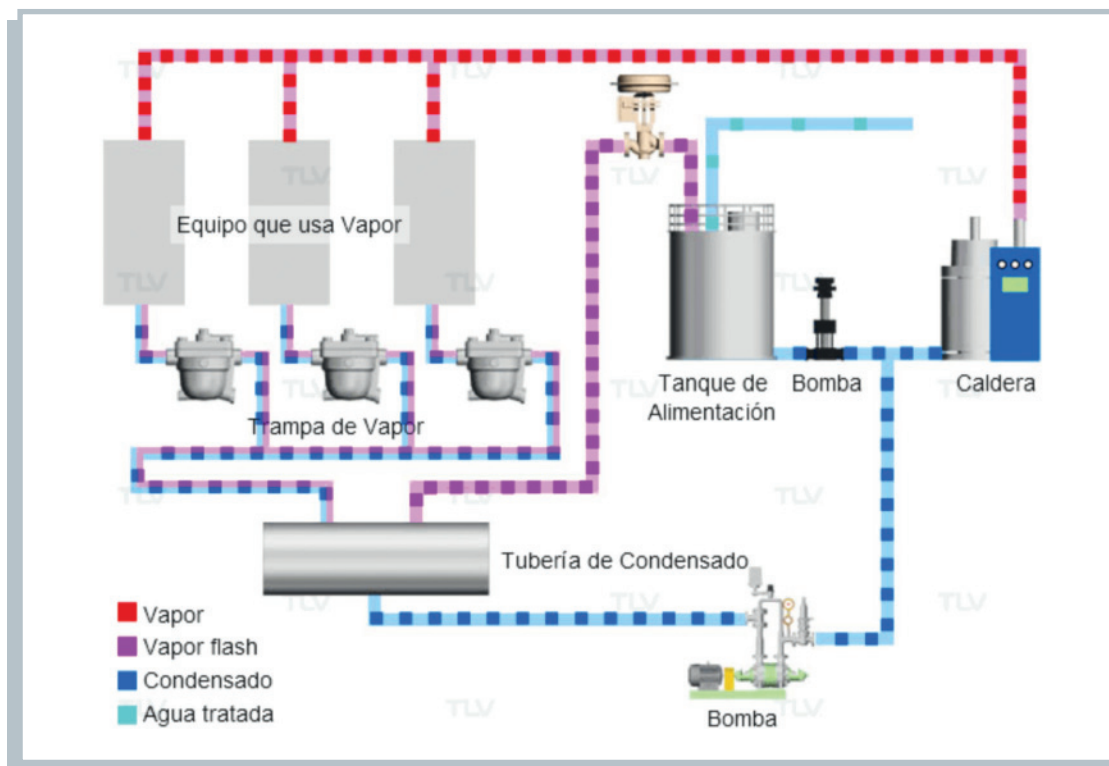
Ilustración 13. Instalación de calentamiento de aire con recuperación de vapor flash. Fuente: TLV.
