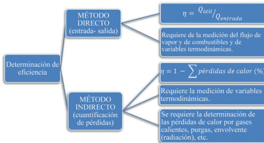
Ilustración 10. Métodos para la determinación de eficiencia de calderas. Fuente: elaboración propia
