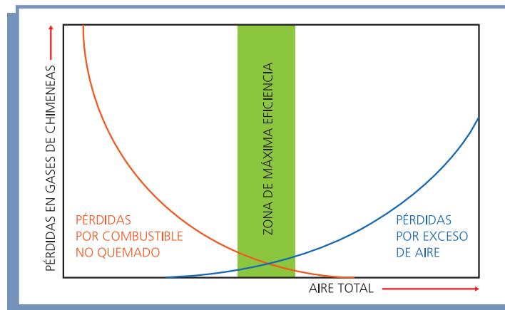
Ilustración 9. Relación entre cantidad de aire y eficiencia. Fuente: CONUEE. Bases para el ahorro de calderas y sistemas de vapor
