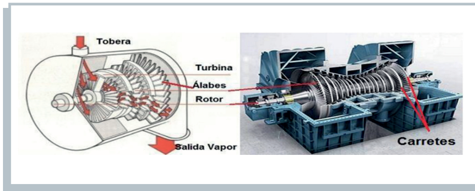
Ilustración 18. Turbina de vapor.
