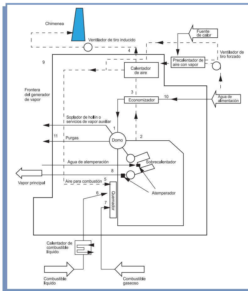
Ilustración 26. Diagrama Simplificado del Generador de Vapor. Fuente: "Eficiencia Energética en la Generación y Distribución del Vapor", Colciencias Colombia, Libertad y Orden UPME.
