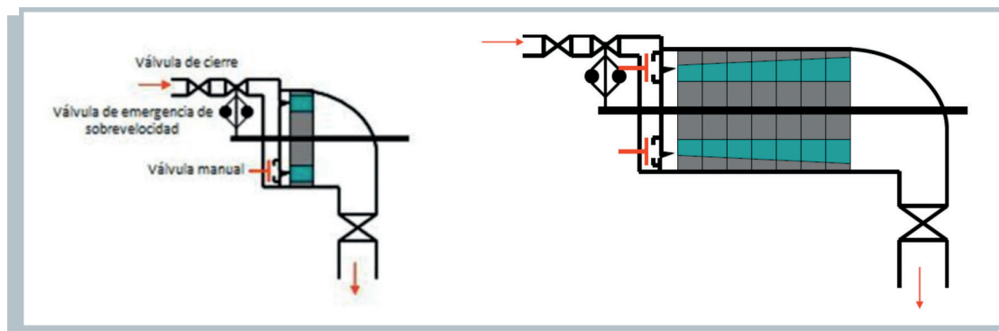
Ilustración 19. TV a contrapresión mono - etapa y multietapas.
