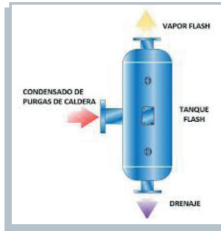
Ilustración 12. Separador de vapor flash. Fuente: Tesis ingeniería mecánica, Universidad Cesar Vallejos 2015.
