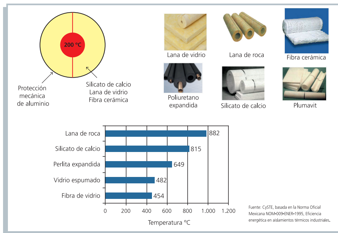
Ilustración 16 Materiales aislantes
