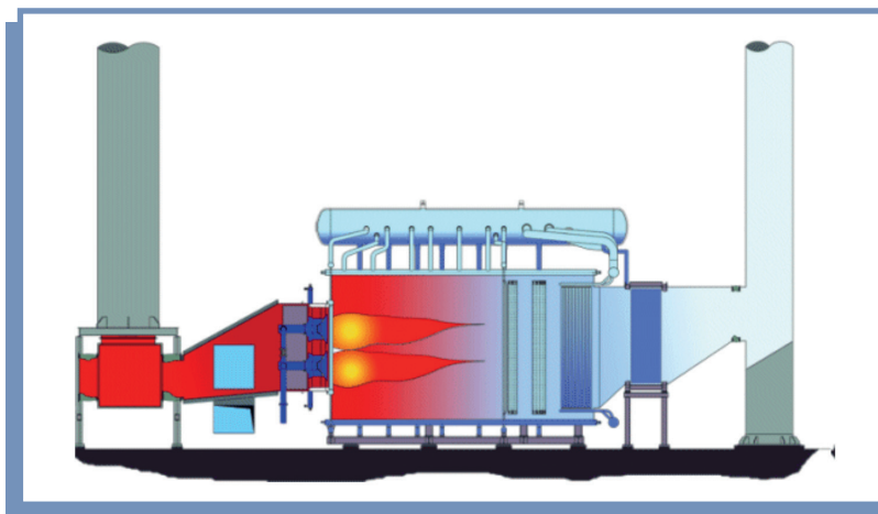
Ilustración 7. Esquema - Caldera HRSG (horizontal). Fuente: Curso - Centrales Térmicas de Ciclo Combinado (renovetc)
