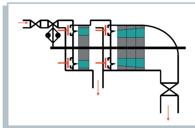
Ilustración 21. TV de extracción. Fuente: US DOE Steam BestPractices End User Training.
