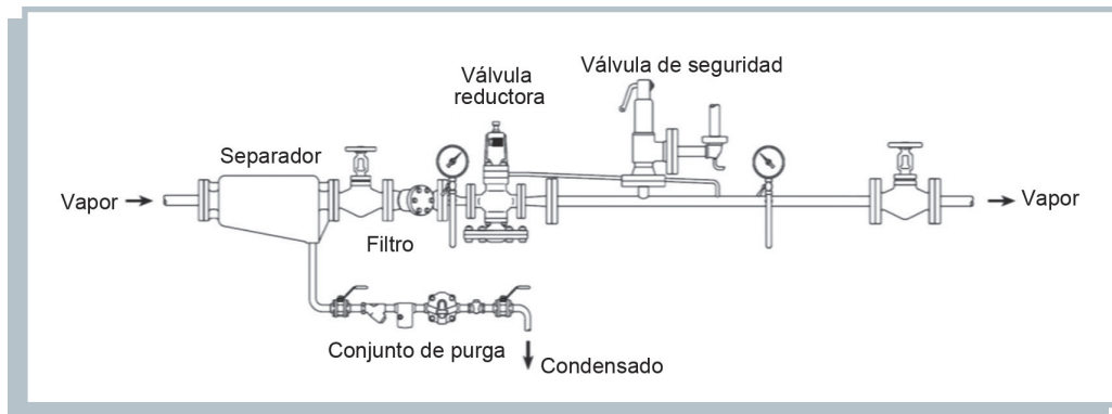
Ilustración 22. Estación de válvula reductora de presión. Fuente: Spirax Sarco.
