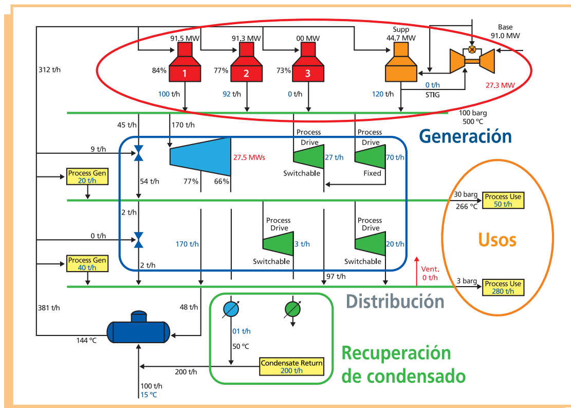
Ilustración 2. Esquema de una red de vapor. Fuente: elaboración propia
