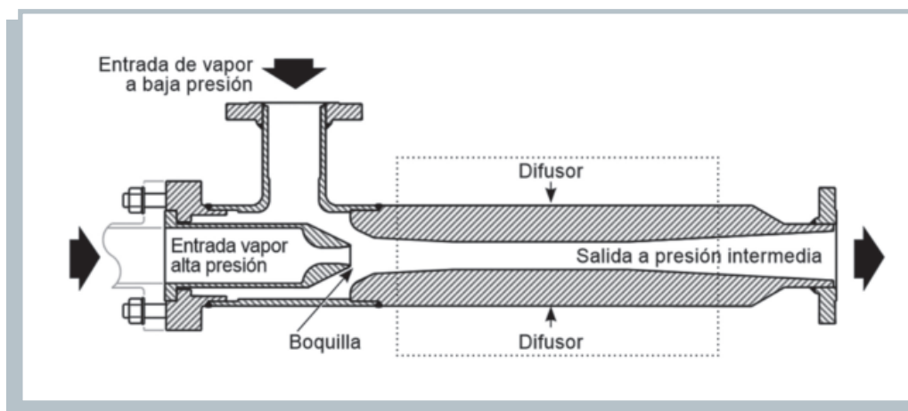
Ilustración 23. Esquema de un termocompresor. Fuente: Spirax Sarco, 2017.
