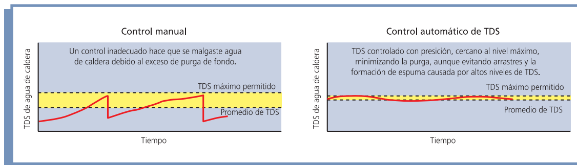
Ilustración 11. Comparación de tipos de control de purgas. Fuente: Spirax Sarco
